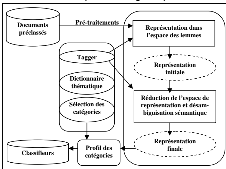
Figure 1 : Principe de construction des classifieurs
